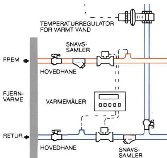
Principskitse
